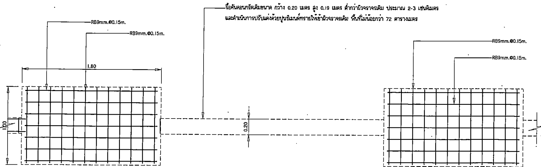
แปลนการวางเหล็ก
