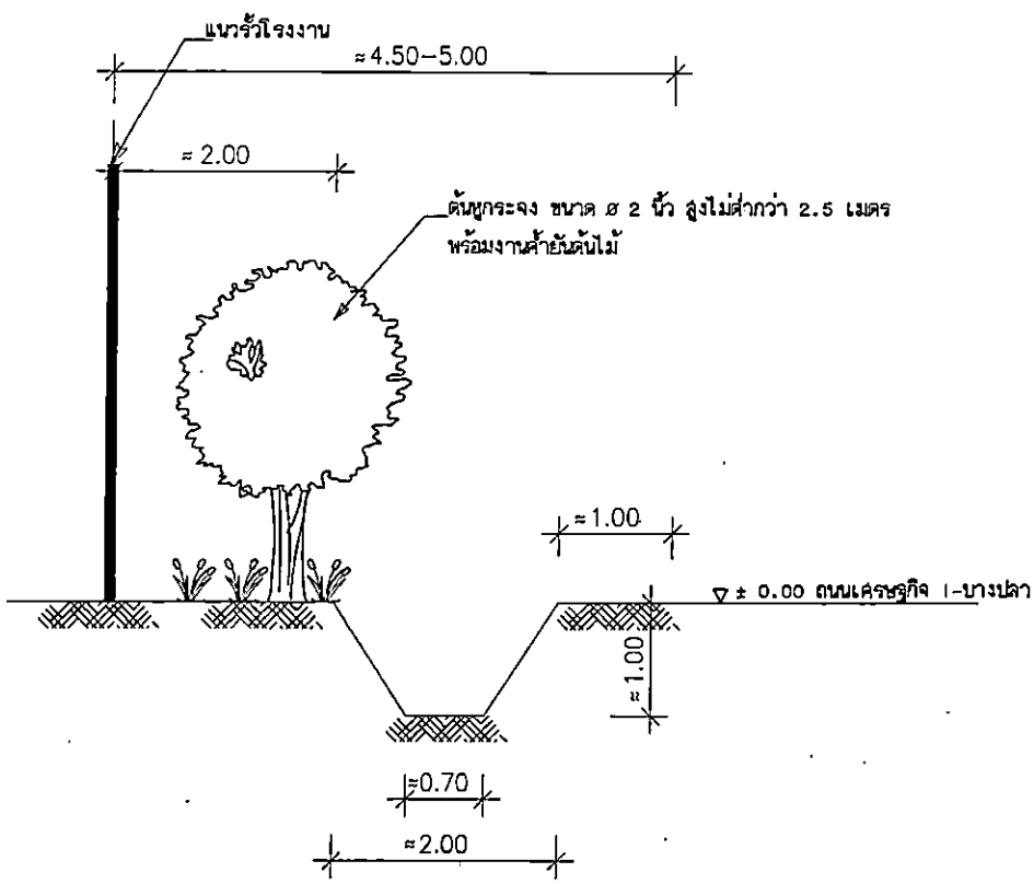
แบบขยายงานปรับปรุงภูมิทัศน์ ZONE 1 งานปรับปรุงภูมิทัศน์ริมถนน 1 ระยะทางไม่ต่ำกว่า 170
