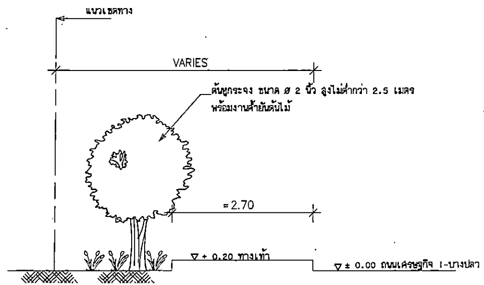
แบบขยายงานปรับปรุงภูมิทัศน์ ZONE 3
