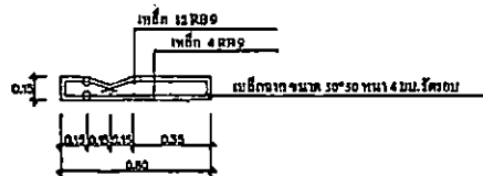
รูปค้ำประตู ค.ส.ล.
