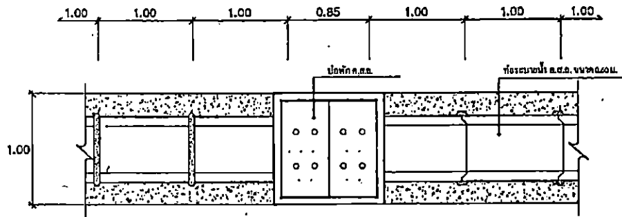
รูปขยายแปลนวางท่อน ค.ส.ล.
