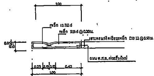
รูปค้ำวางวิ ค.ส.ล.
