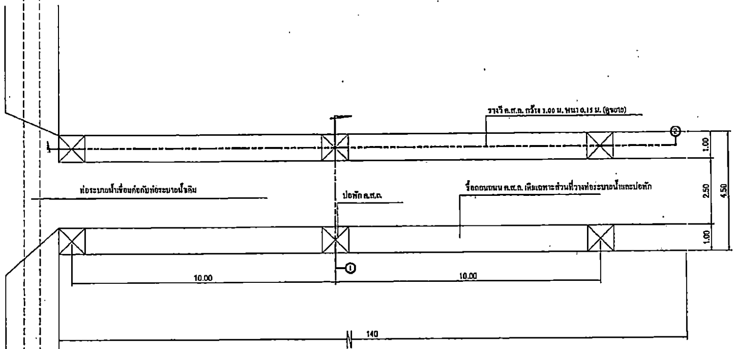
แบบแปลนก่อสร้างถนน วางท่อระบายน้ำ ค.ส.ล.
