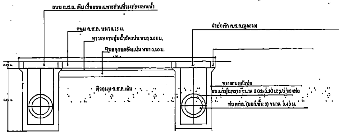
รูปตัดแสดงงานวางท่อ
