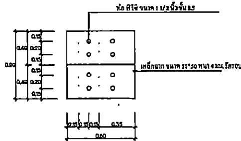
รูปขยายแปลนค้ำประตู ค.ส.ล.
