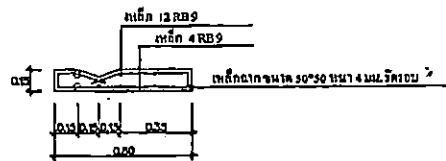
รูปตัดค้ำประตู ค.ส.ท.
