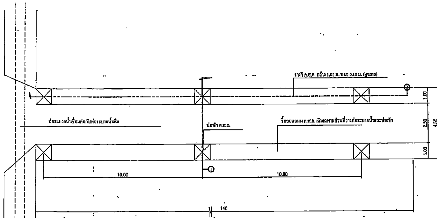
แบบแปลนก่อสร้างถนน วางท่อระบายน้ำ ค.ส.ล.
