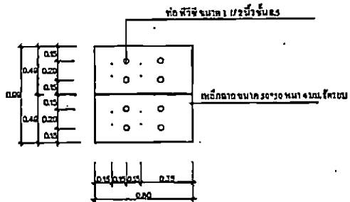
รูปขยายแปลนค้ำประตู ค.ส.ท.
