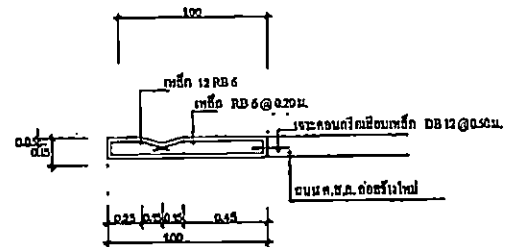
รูปตัดขวางวิ ค.ส.ท.
