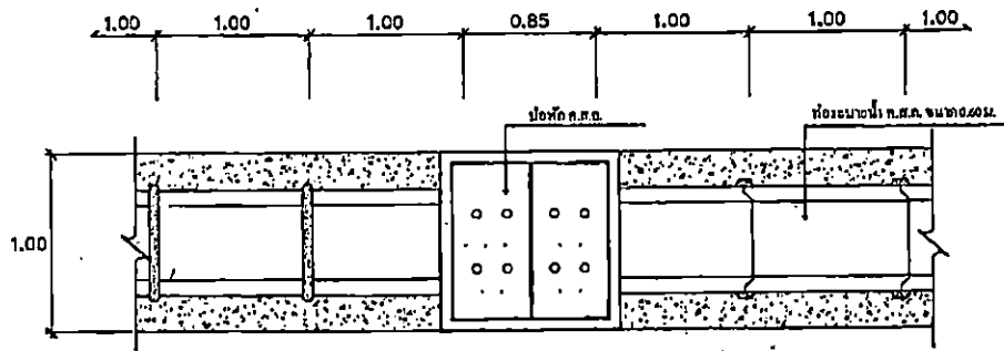
รูปขยายแปลนวางท่อน ค.ส.ท.
