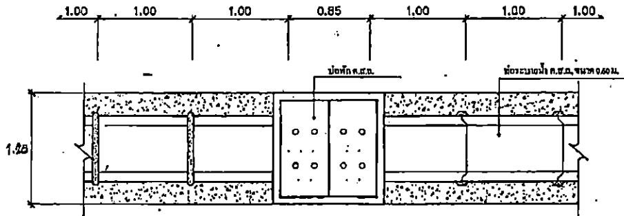
รูปขยายแปลนวางท่อ ค.ส.ท.
