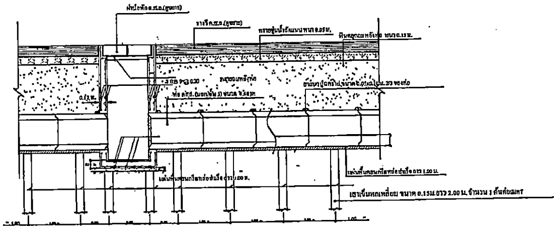
รูปตัดตามยาว
