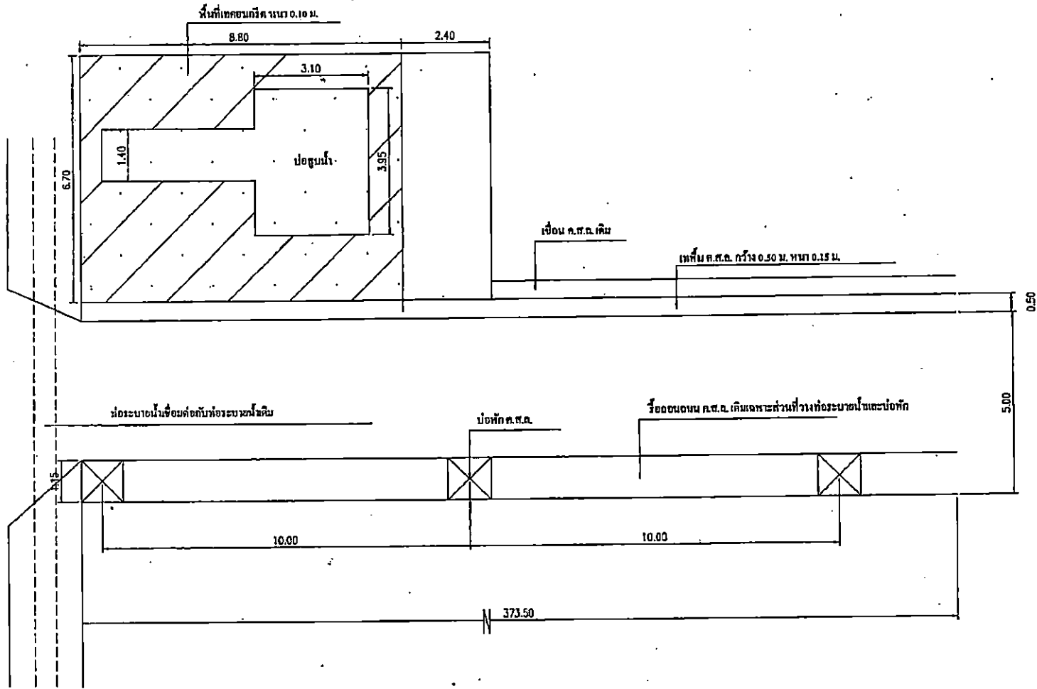
แบบแปลนวางท่อระบายน้ำ ค.ส.ล.
