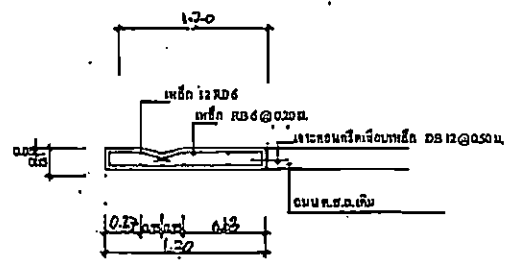
รูปตัดค้ำวาง ค.ส.ท.
