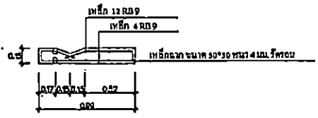
รูปตัดค้ำปัดหัก ค.ส.ท.
