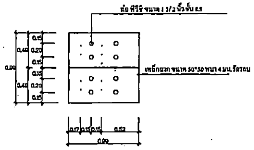
รูปขยายแปลนค้ำปัดหัก ค.ส.ท.
