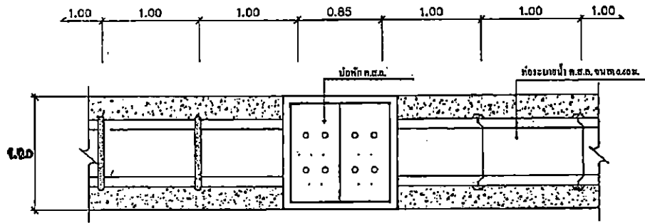
รูปขยายแปลนวางท่อ ค.ส.ล.
