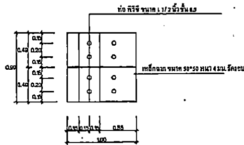
รูปขยายแปลนผ่านบ่อพัก ค.ส.ล.
