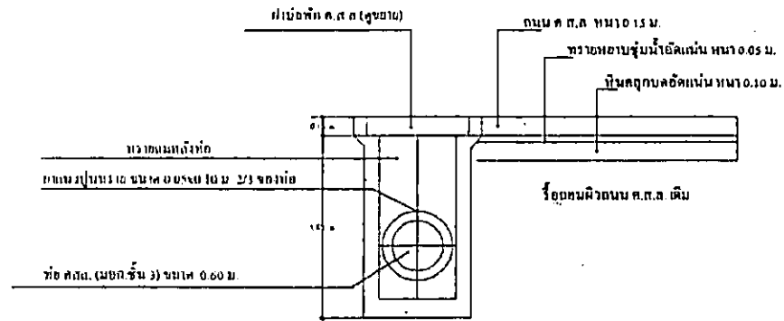
รูปตัดแสดงงานวางท่อ 1
