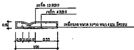
รูปตัดผ่านบ่อพัก ค.ส.ล.
