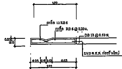
รูปตัดวางวิ ค.ส.ล.
