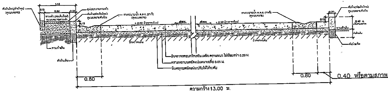
รูปตัด ①-① (ช่วงถนนที่ 1-2 ระยะที่ 0.00 - 267.00 เมตร)
