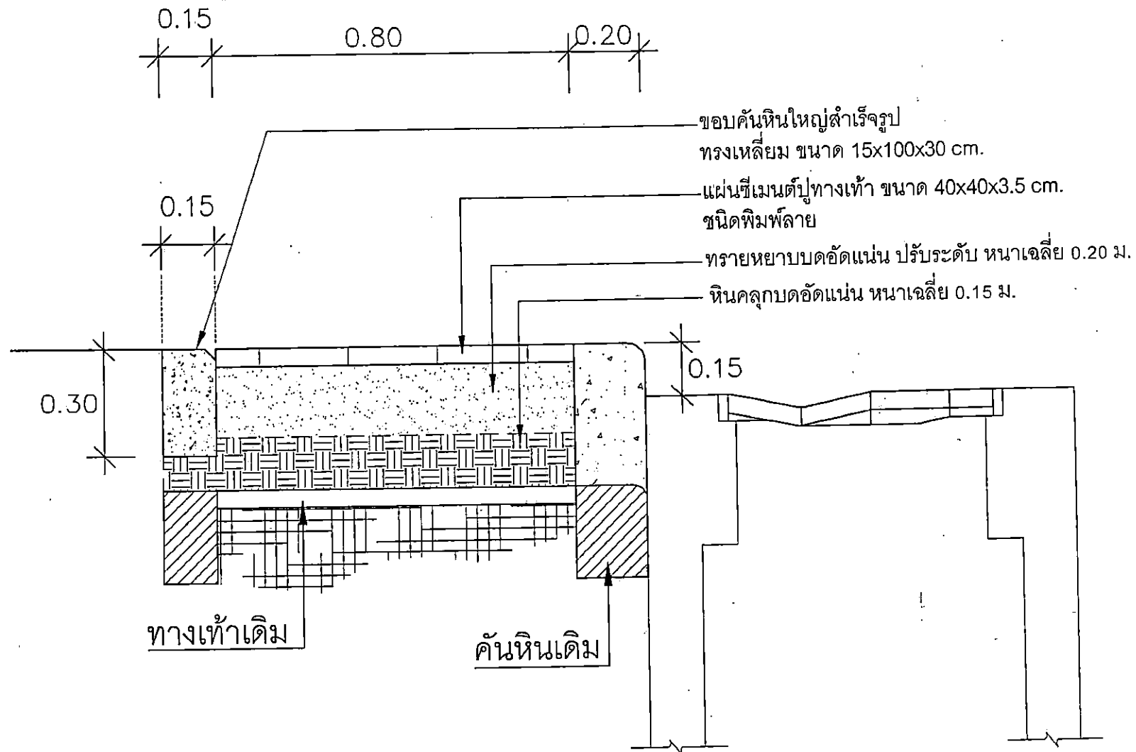
แบบขยายทางเท้า
