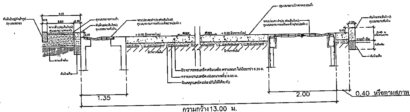
รูปตัด ②-② (ช่วงถนนที่ 1 ระยะที่ 0.00 - 175.00 เมตร)
