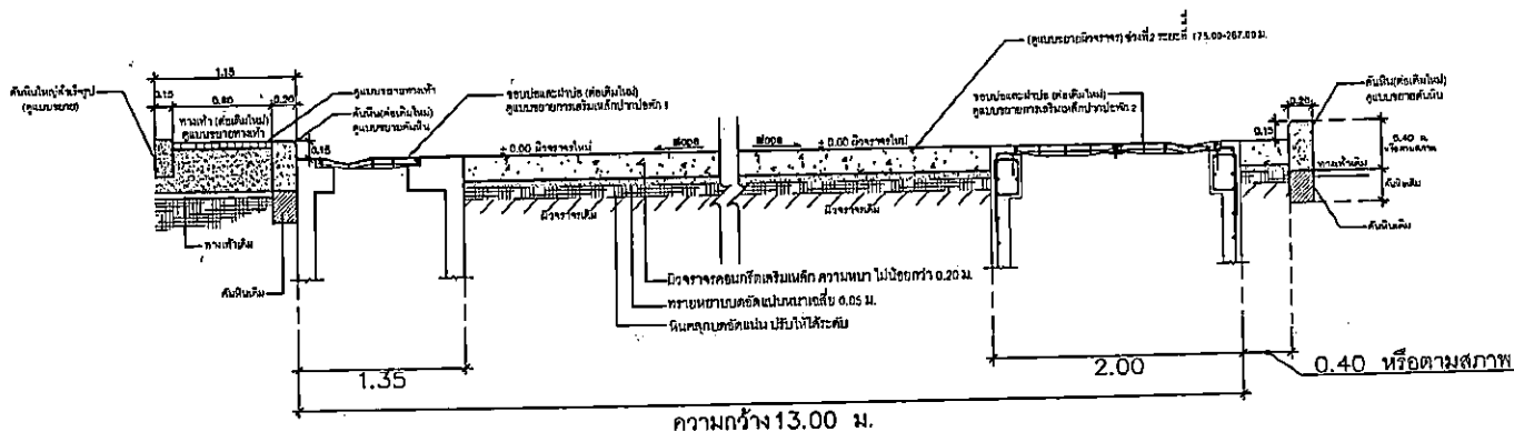
รูปตัด (ช่วงถนนที่ 2 ระยะที่ 175.00 - 267.00 เมตร)
