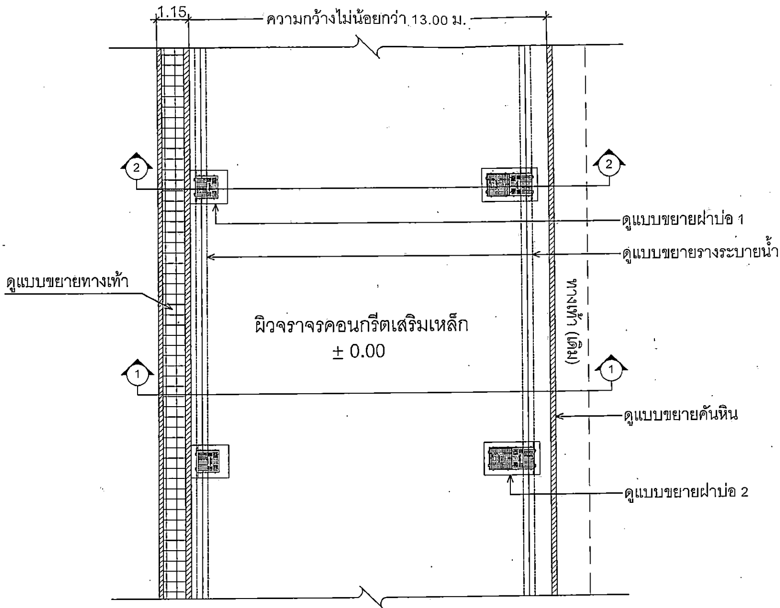
แปลนปรับปรุงขยายฝัวจราจรร ฝาบ่อ คั่นหิน ทางเท้า และรางระบายน้ำ
