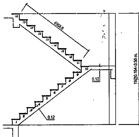
รายละเอียดบันได ST1 Scale 1:50
