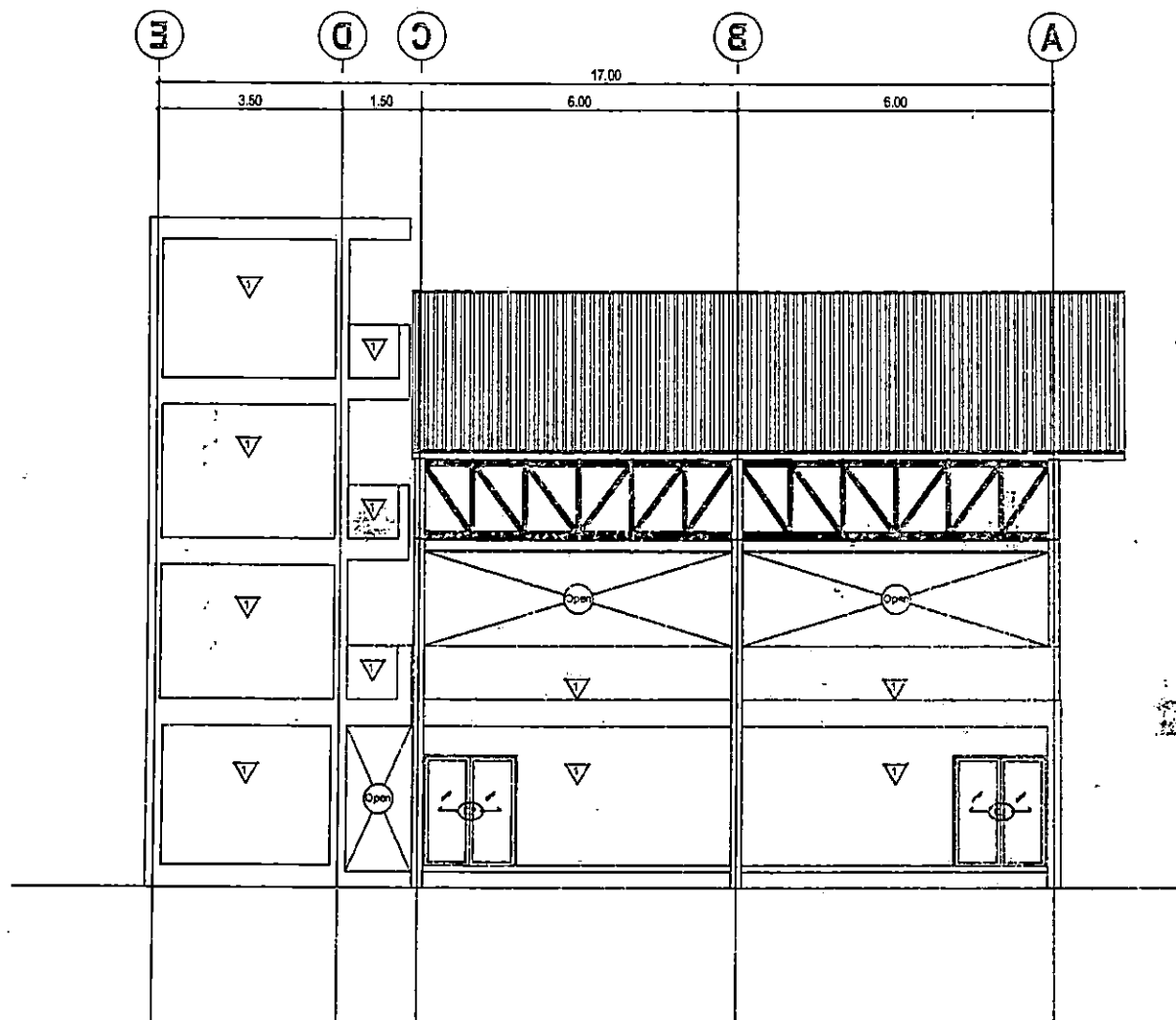
รูปด้านซ้ายอาคาร Scale 1:100
