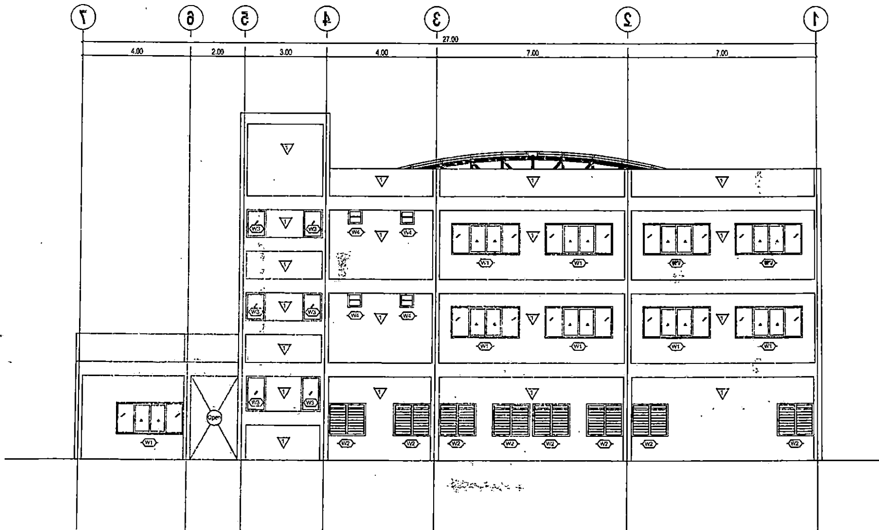
รูปด้านหลังอาคาร Scale 1:100
