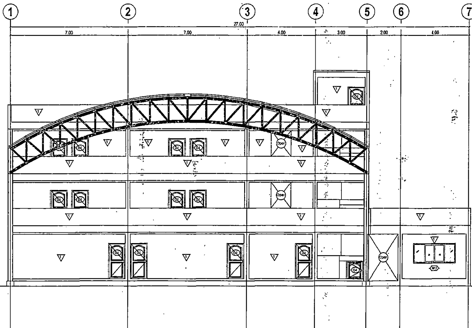
รูปด้านหน้าอาคาร Scale 1:100
