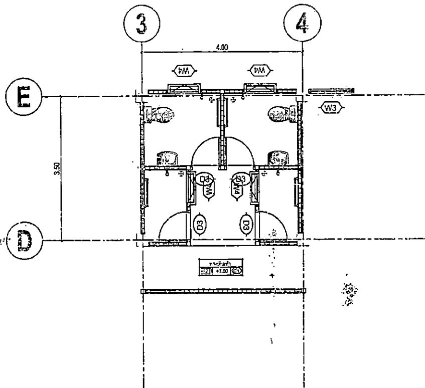
แบบขยายห้องน้ำ 1 ชั้น 2, 3
